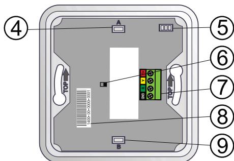
Slika 2: 4 – A taster, 5 – LED indikator, 6 – Kontakt za sabotažu, 7 – priključci magistrale, 8 – Proizvodna šifra, 9 – B taster
