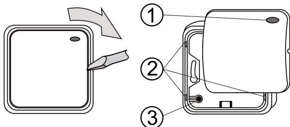
Slika: 1 – Maska LED indikatora, 2 – Plastični jezičci osnovne, 3 – Stalni magnet
